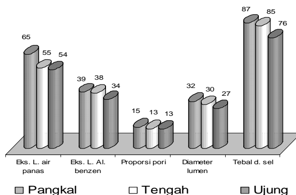
Gambar 7. Perbandingan Bambu Atas Dasar Bagian Batang Menurut Ekstraktif Larut Air Panas (%), Ekstraktif Larut Alkohol Benzen (%), Proporsi Sel Pori (%), Diameter Rongga Sel Serat (Mikron), dan Tebal Dinding Sel Serat (Mikron).
