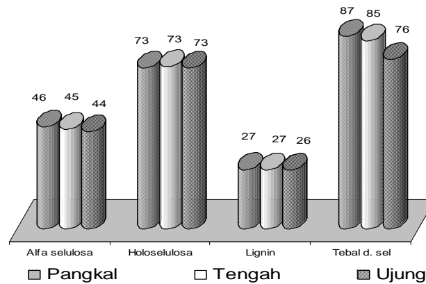
Gambar 6. Perbandingan Bamboo Atas Dasar Bagian Batang Menurut Alfa Selulosa (%), Holoselulosa (%), Lignin (%), dan Tebal Dinding Sel Serat (Mikron). Keterangan : Nilai Tebal Dinding Sel Serat Dikalikan 0,001
