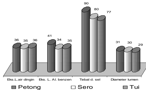
Gambar 4. Perbandingan Bambu Atas Dasar Jenis Menurut Ekstraktif Larut Air Dingin, Ekstraktif Larut Alkohol Benzen (%), Tebal Dinding Sel Serat (Mikron), dan Diameter Lumen Sel Serat (Mikron).
