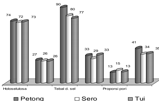
Gambar 5. Perbandingan Bambu Atas Dasar Jenis Menurut Holoselulosa (%), Lignin (%), Tebal Dinding Sel Serat (Mikron), Proporsi Sel Serat (%), Proporsi Sel Pori (%), dan Ekstraktif Larut Alkohol Benzen (%).
