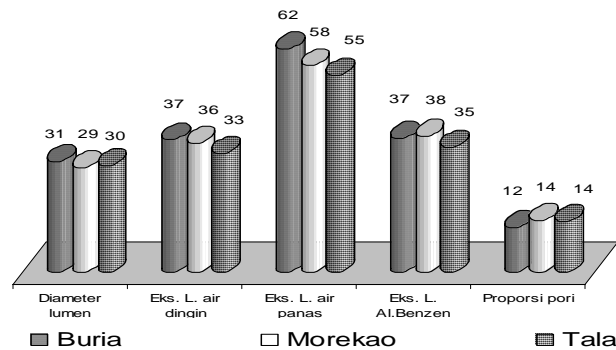
Gambar 2. Perbandingan Bambu Atas Dasar Lokasi Menurut Diameter Lumen (Mikron), Ekstraktif Larut Air Dingin (%), Ekstraktif Larut Air Panas (%), Ekstraktif Larut Alkohol Benzen (%), dan Proporsi Sel Pori (%).
